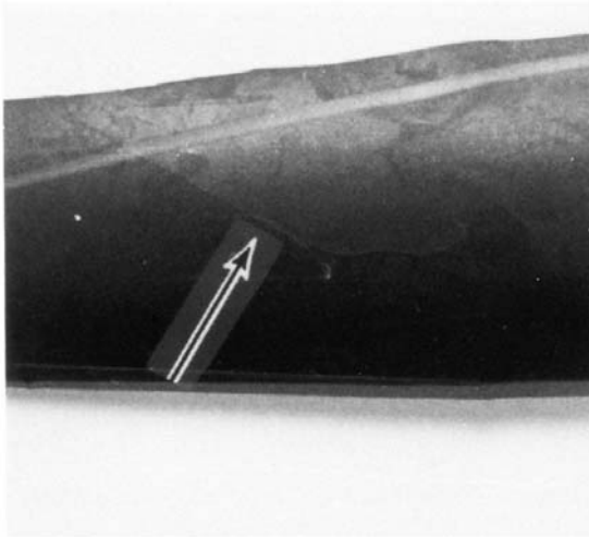
FIG. 15 Mold Marks
