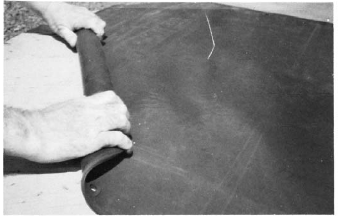
FIG. 29 Blanket Rolling
